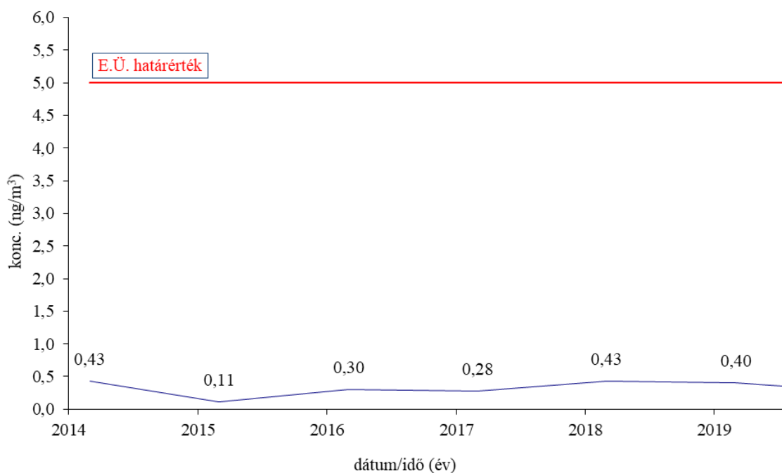
kadmium/ PM 10 éves átlagkoncentráció alakulása 2014. és 2019. között az indikatív mérőponton
