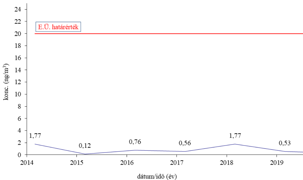
39. ábra: nikkel/PM 10 éves átlagok az időszakos indikatív mérések eredményei alapján 2014-2019. között.
